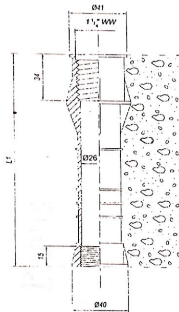
TYPE CS1
