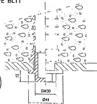
TYPE BLT1
